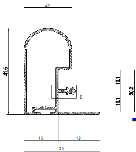
TR025 MANIGLIONE L
