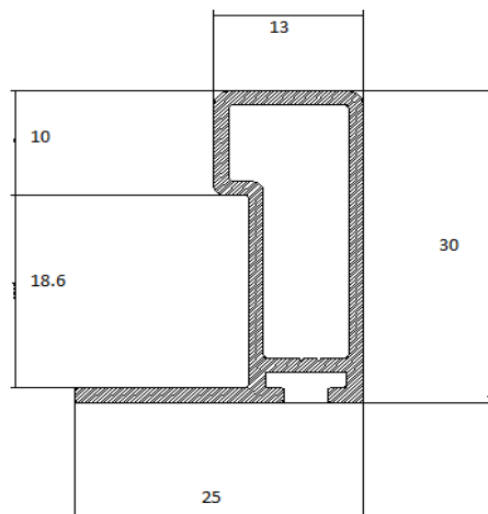
TR021 CONTROMANIGLIA LEGGERA
