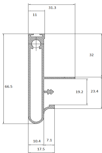
TR014 - MANIGLIONE STONDATO LARGO 66 PER TIRANTE CON MASCHI PANNELLO 18
