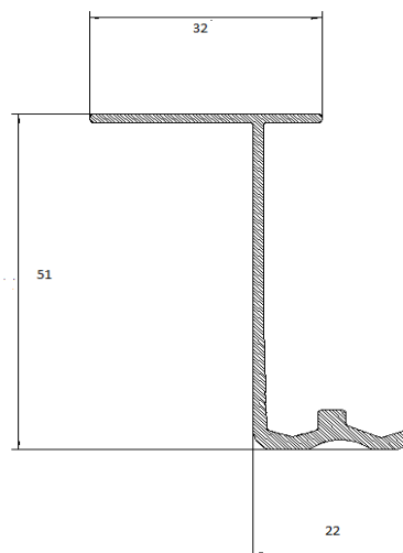
TR005 - BINARIO SUPERIORE RAM
