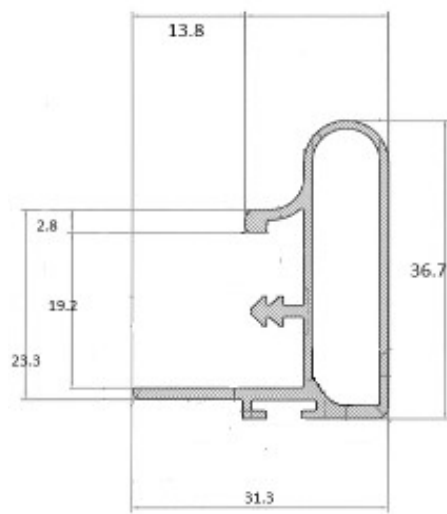
TR023 - MANIGLIONE QUADRATO PER TIRANTE CON MASCHI PANNELLO 18
