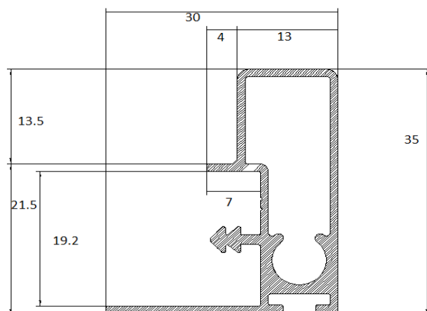
TR023 - MANIGLIONE QUADRATO PER TIRANTE CON MASCHI PANNELLO 18
