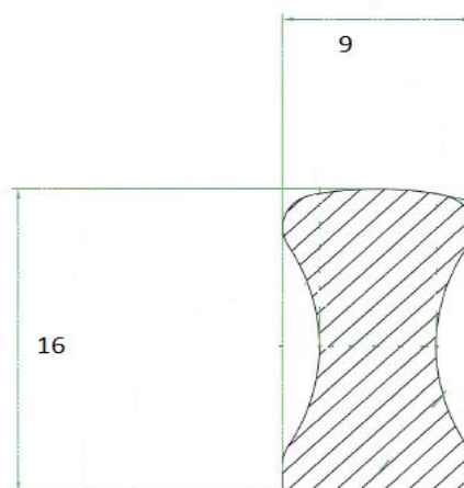
TR012 MANIGLIA CLESSIDRA 16X9
