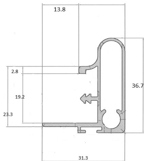
TR014 - MANIGLIONE STONDATO LARGO 66 PER TIRANTE CON MASCHI PANNELLO 18
