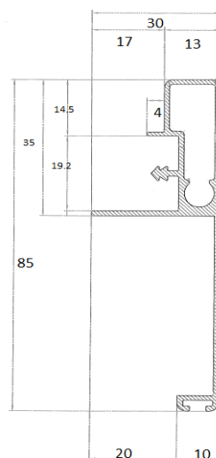
TR026/B - MANIGLIONE QUADRATO LARGO PER TIRANTE CON MASCHIO 85 PER PANNELLO 18
