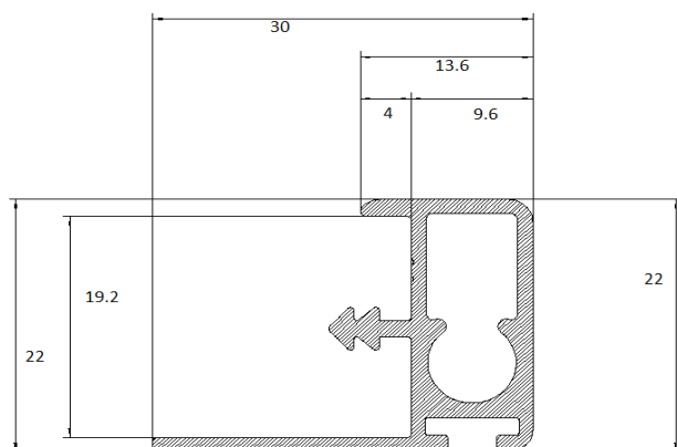
TR024 - CONTROMANIGLIONE PER TIRANTE PER PANNELLO 18
