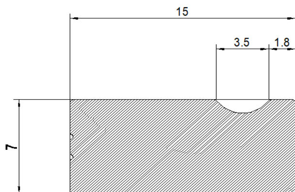
TR012 MANIGLIA RETTANGOLARE 15X7
