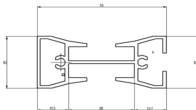
TR027 - PROFILO MONTANTE CABINA ARMADIO
